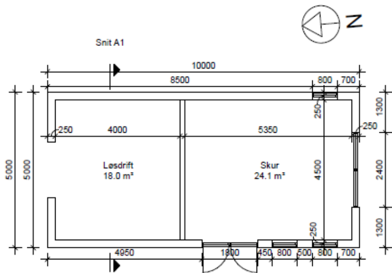
Snit A1 Plantegning - 1:100
