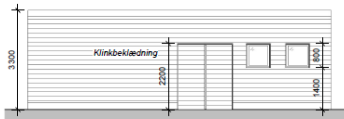
Østfacade - 1:100
