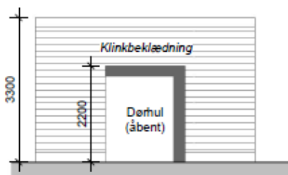
Sydfacade - 1:100
