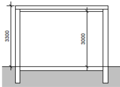
Snit A1 - 1:100
