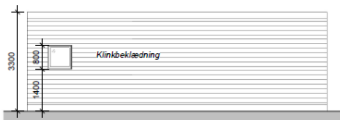
Vestfacade - 1:100
