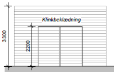
Nordfacade - 1:100
